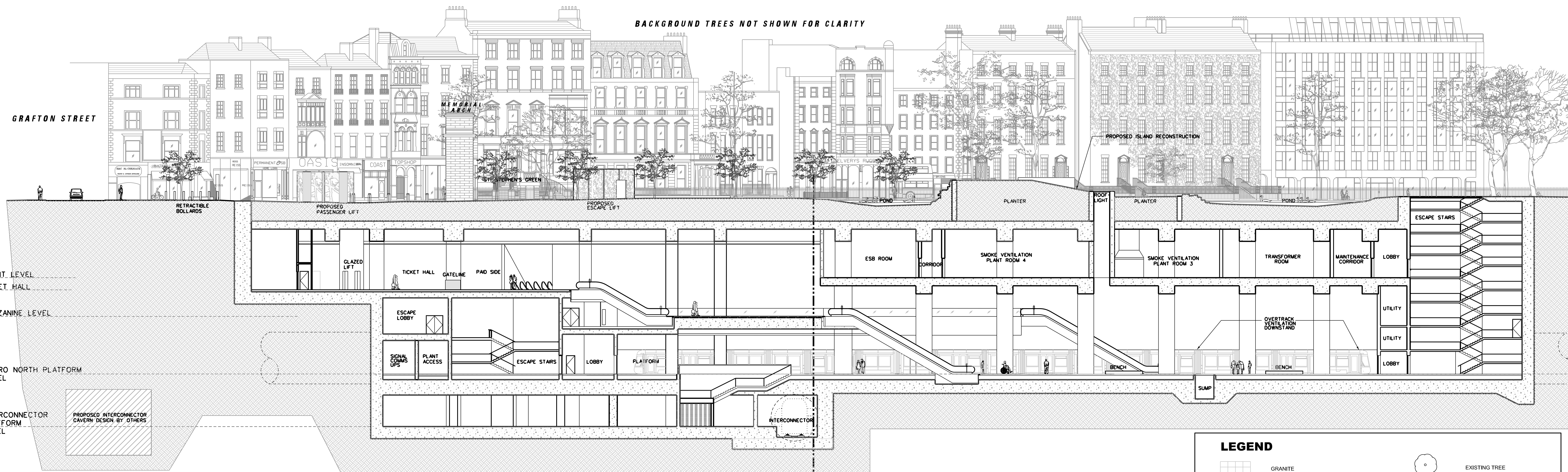
LONGITUDINAL SECTION A-A SCALE 1:200
