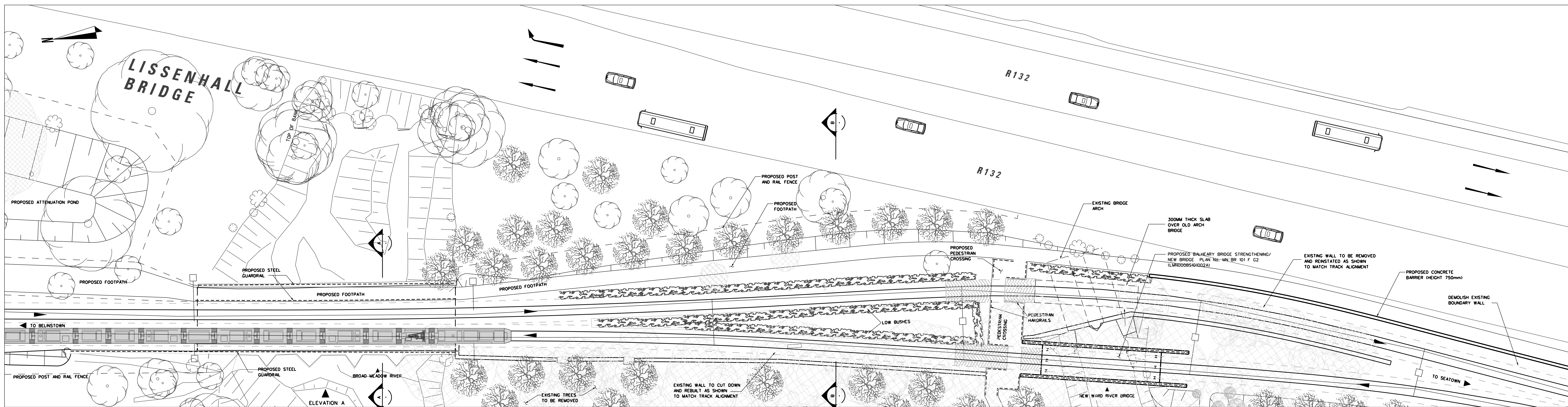
PLAN SCALE: 1:200
